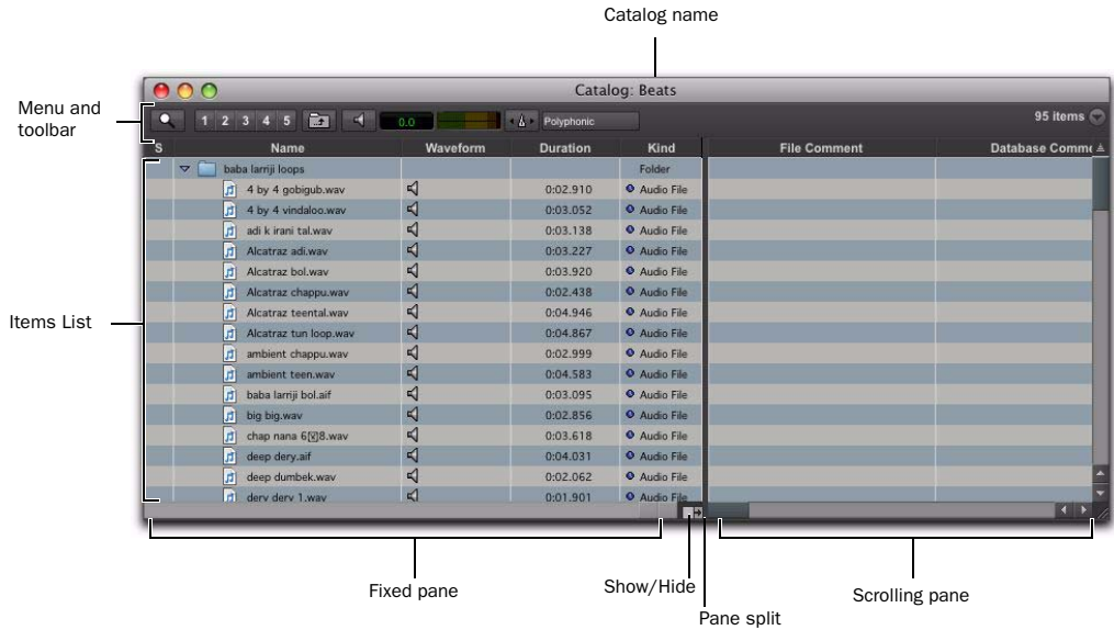
Catalog browser
